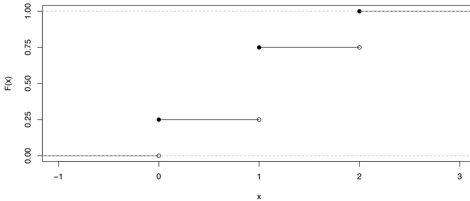
Verteilungsfunktion
