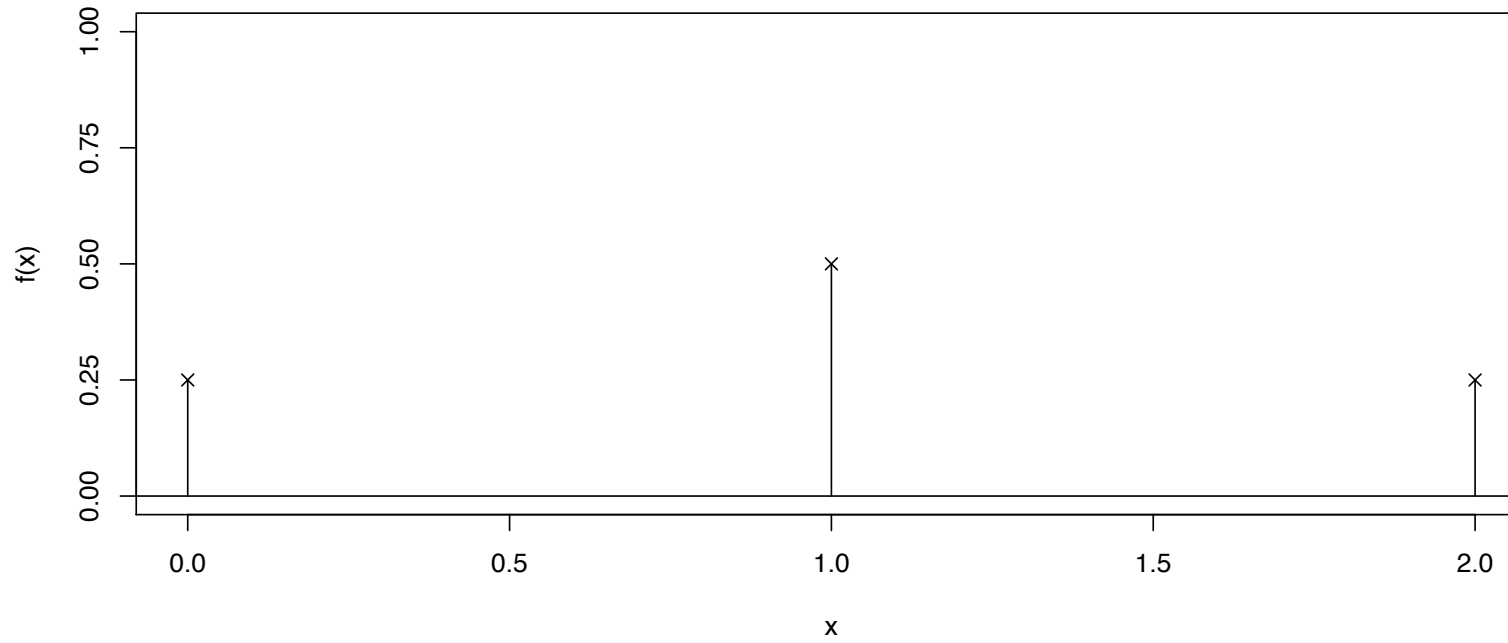
Wahrscheinlichkeitsfunktion
